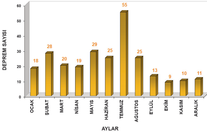
2017 YILI TÜRKİYE VE YAKIN ÇEVRESİ DEPREM HAREKETLİLİĞİ
